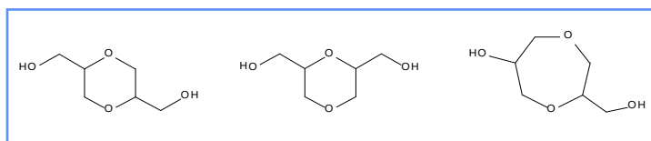
โครงสร้าง Cyclic-glycerine (Cyclic-glycerol)
